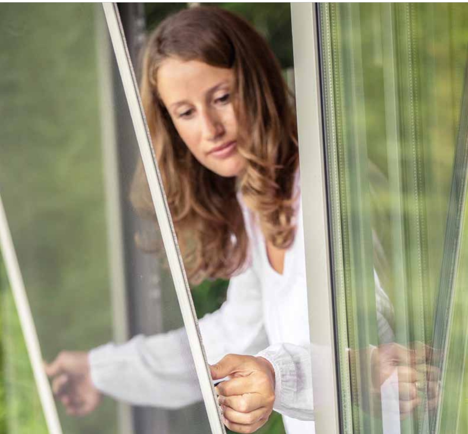
34 mm Spannrahmen mit Bürstendichtung, einfaches Aushängen mit gefederten Einhängewinkeln, maximale Größe 200x250 cm, 24 mm Mittelsprosse ab 180 cm Höhe.
