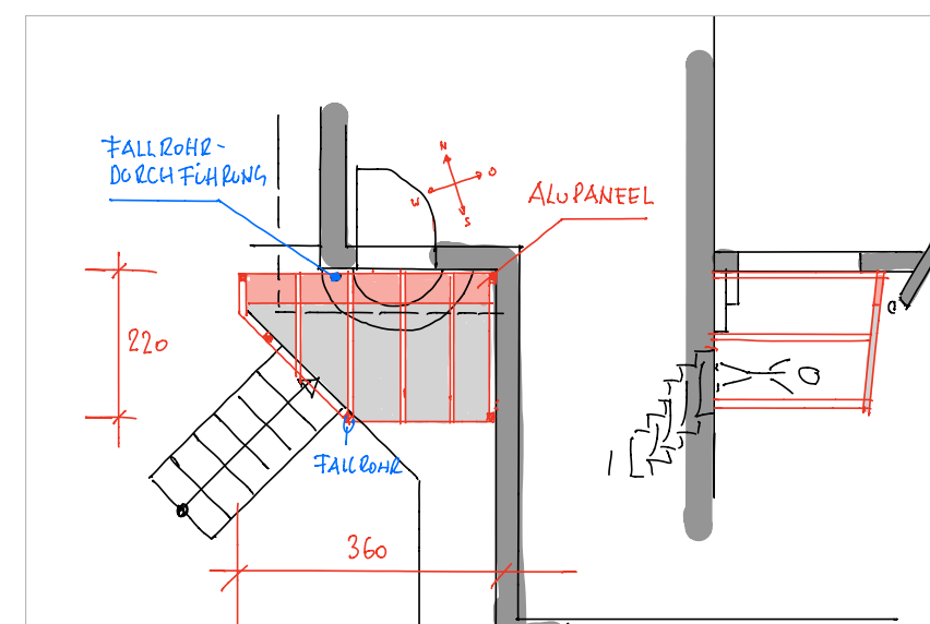
Entwurfsskizze
